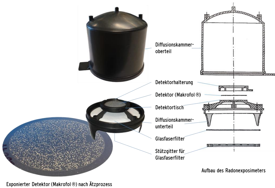
Abbildung 3-3 Bauweise des BfS-Festkörperspurdetektors
